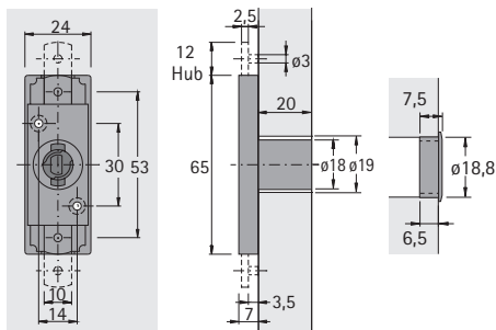
Zylinder-Schubstangenschloss
