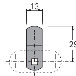
Riegel gekröpft
