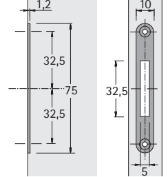
Riegel flach
