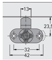
Zylinder-Hebelschloss
