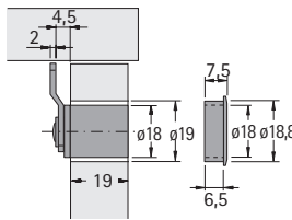
Riegel gekröpft
