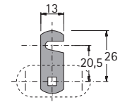
Riegel flach
