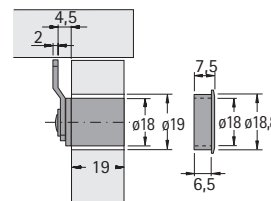
Riegel gekröpft
