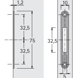
Riegel flach
