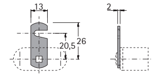
Riegel flach
