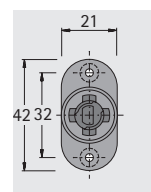
Zylinder-Druckschloss
