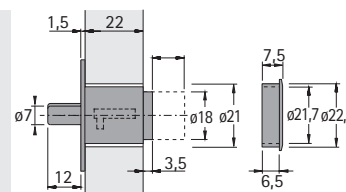
Zylinder-Druckschloss
