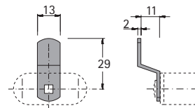
Riegel gekröpft
